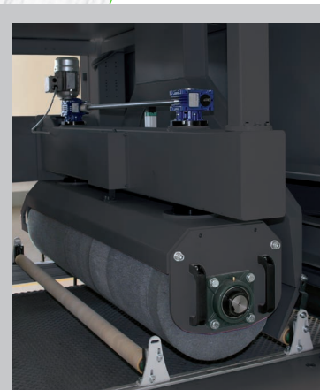
Gruppo spazzola longitudinale Longitudinal brush unit Groupe brosse longitudinale
