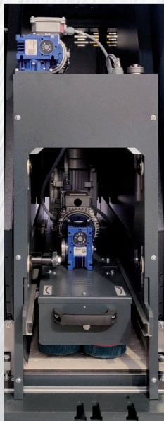
Gruppo spazzole tangenziali Tangential brushes unit Groupe de brosses système tangential
