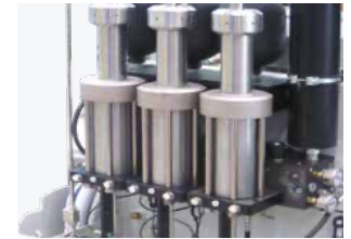
Multiplicadores de presión
